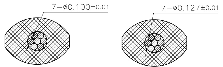
SECTION A-A (4:1) SECTION A-A (4:1)
