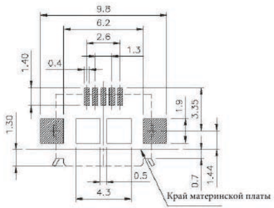
План монтажа
